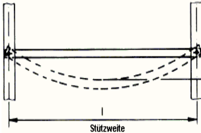
Abb. 1: Höchstzulässige Durchbiegung der tragenden Elemente von Lagereinrichtungen
