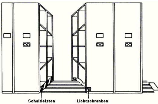
Abb. 14: Sicherung durch Schaltleisten oder Lichtschranken
